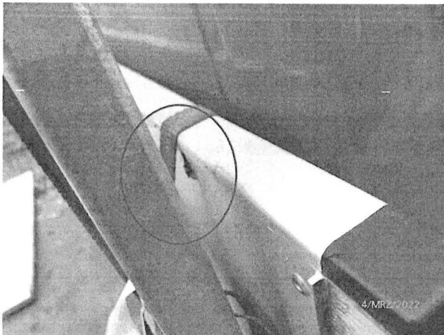
Schutzgitter am Befestigungspunkt Bordwand vorn ausgerissen
