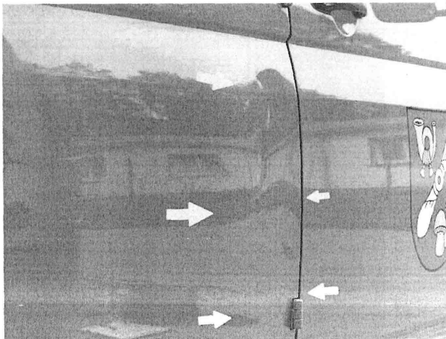
Tür hr ein-/ und durchgedrückt, geknickt
