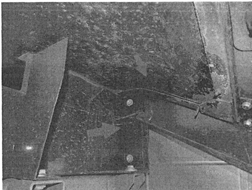
Pritschenrahmen geknickt
