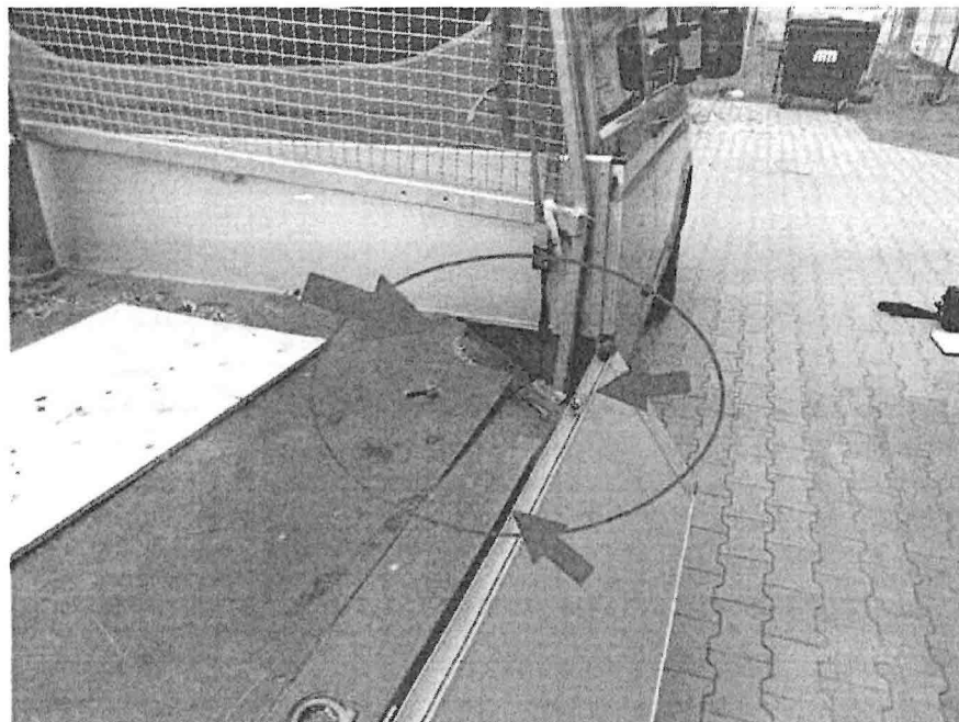
Pritschenboden gebrochen, Rahmen Pritschenrahmen geknickt
