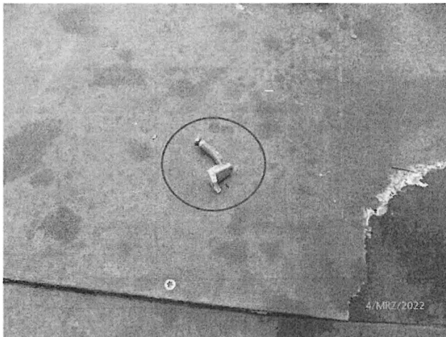
Scharnier Bordwand rechts vorn ausgerissen/ gebrochen
